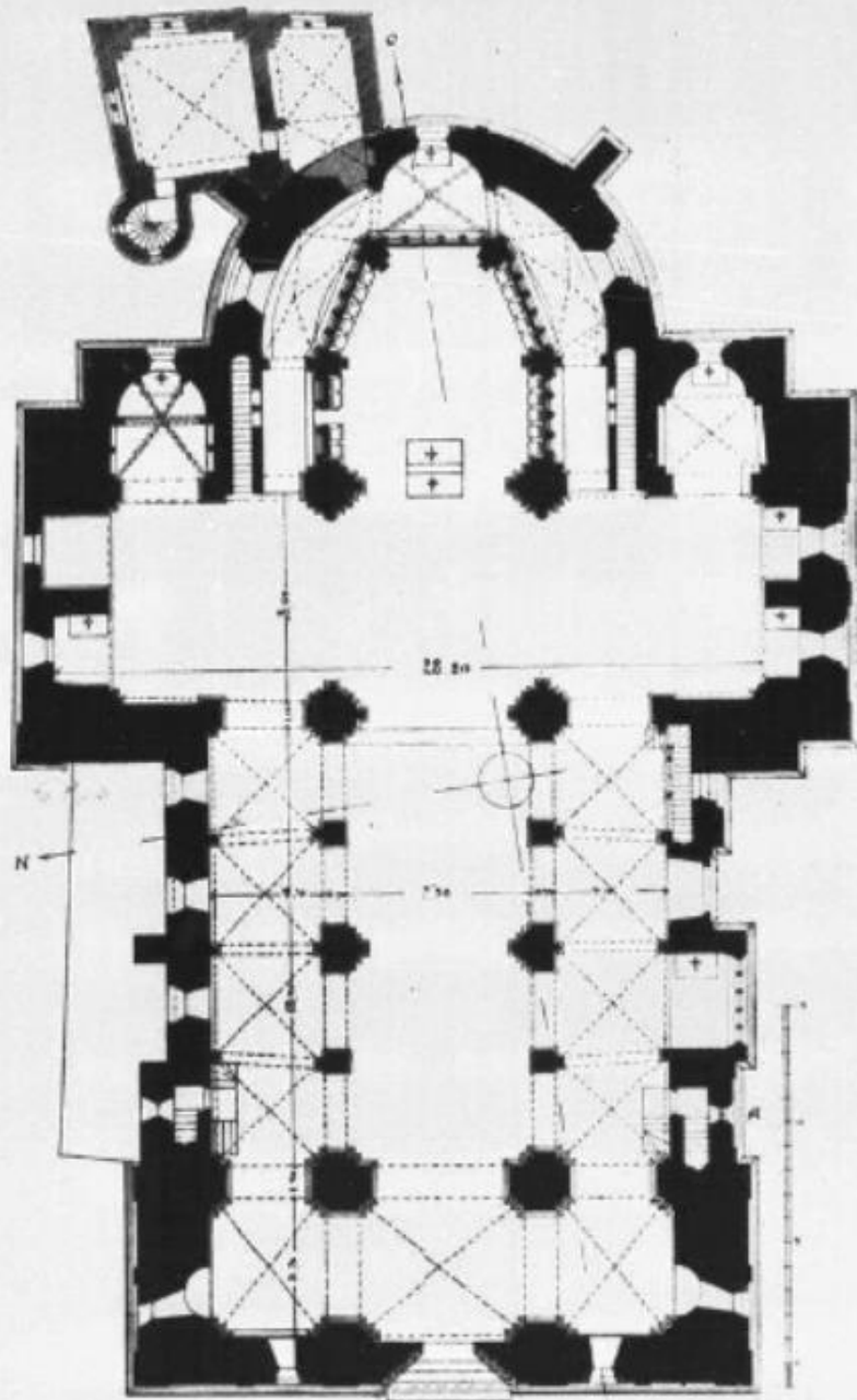
Fig. 63. Limburg. Südkirche St. Georg. Erdgeschoss-Grundriss.
