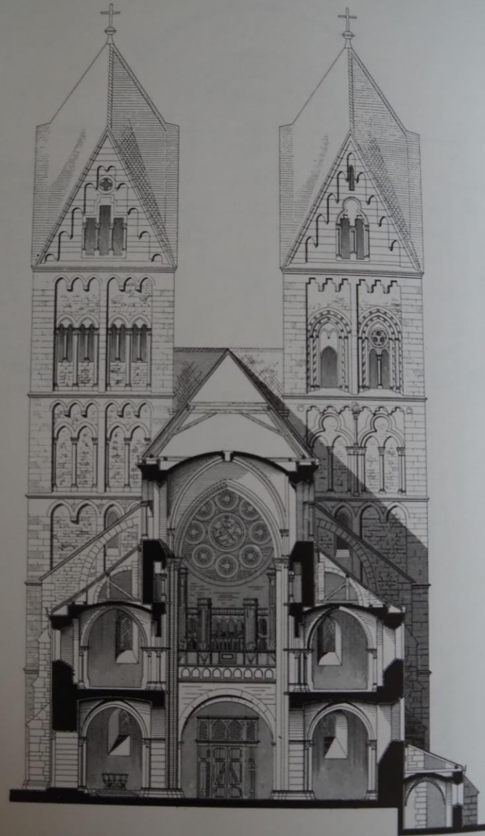
Querschnitt durch das Langhaus (A. Cremer nach H. Stier), M. 1 : 300
